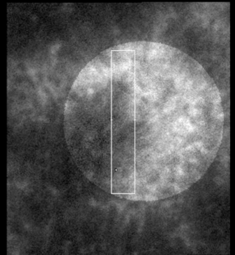
IRIS/SJI Mg
